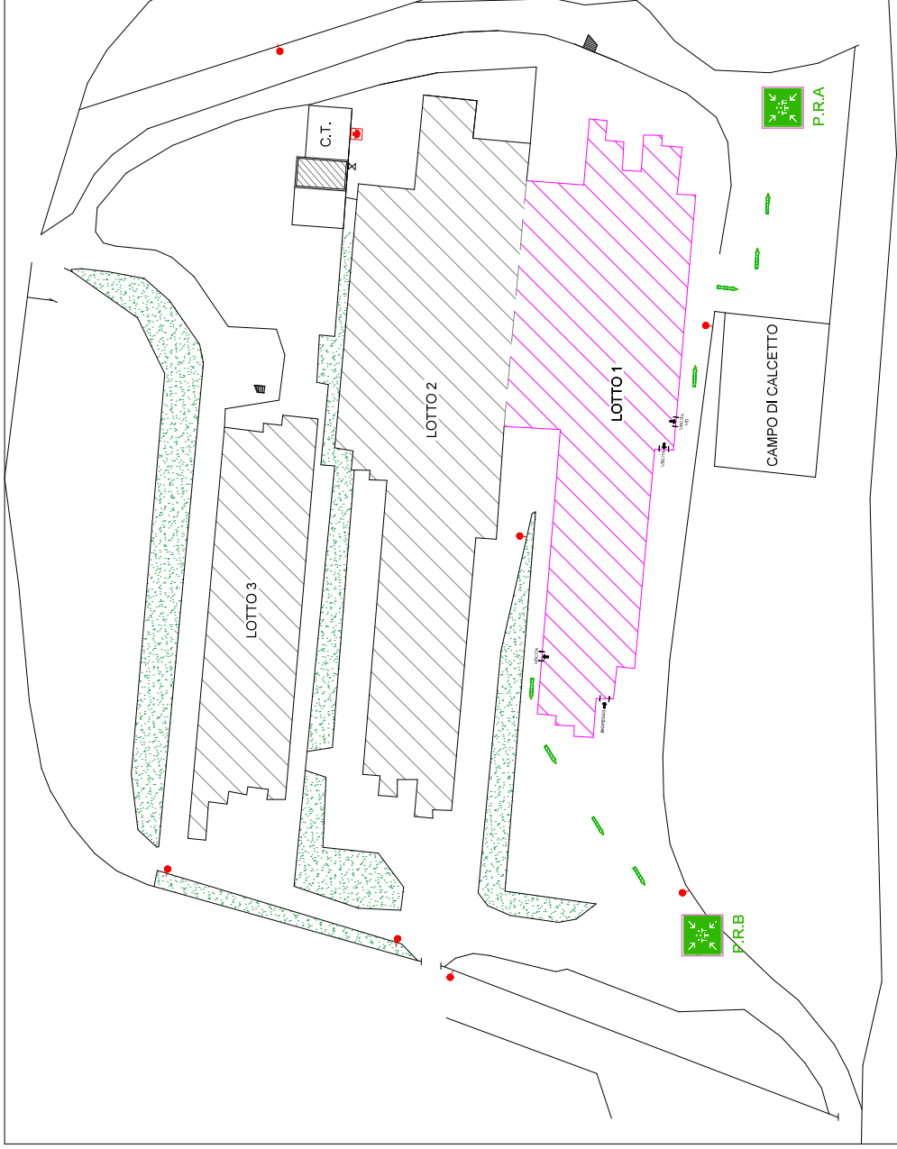
Tavola 0 - Planimetria generale
